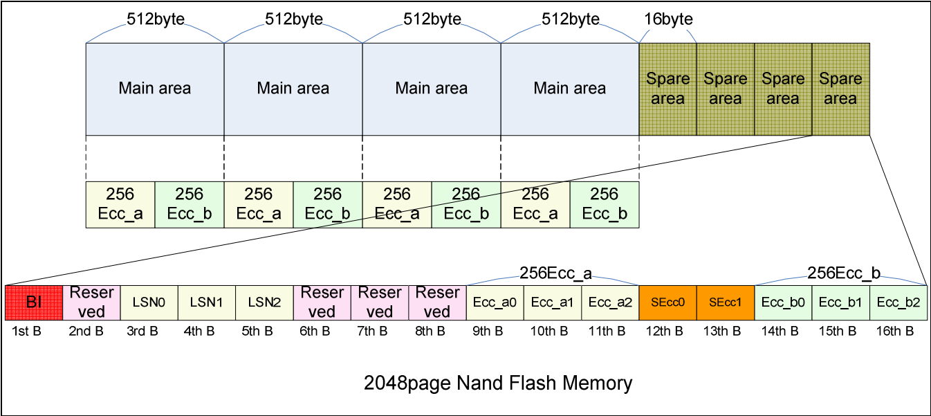
Figure 9-20 SECCSECTOR0~SECCSECTOR7
